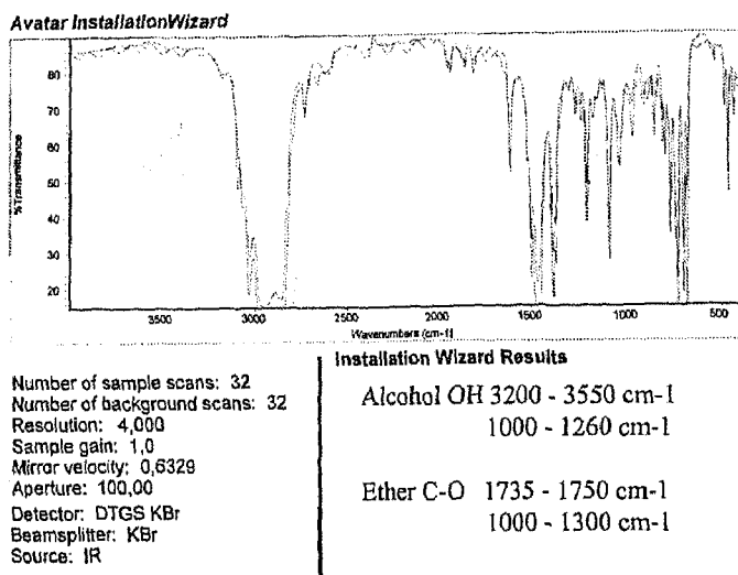
Рис. 2.2. ІЧ-спектр сумішевого бензину з КВД
