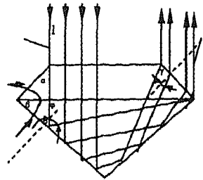
Рис. 5.1. Хід променів в ограненому камені: 1 — промені, що входять, 2 — промені, що виходять
