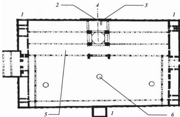
План мечеті в Дамаску:
