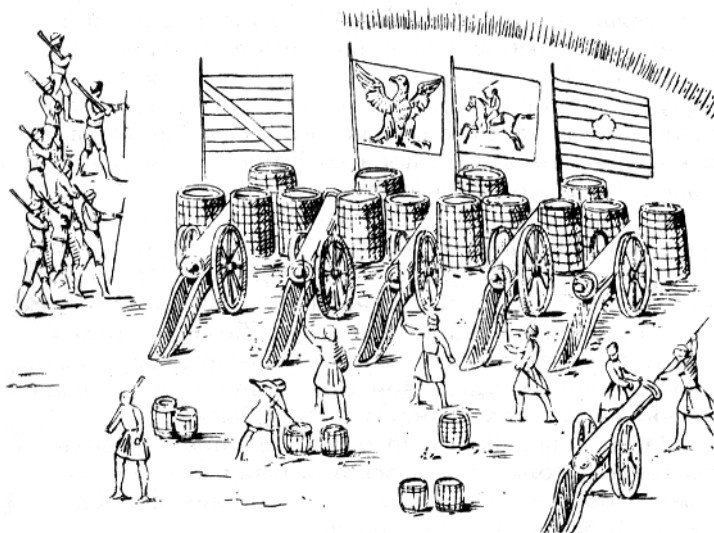
Рис. 10.9. Польська артилерія
